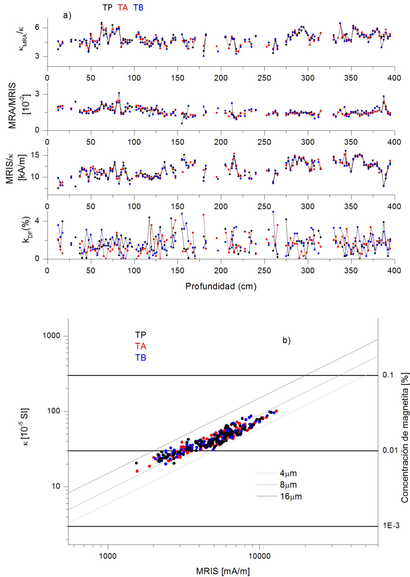
Figura 6. a) Cocientes interparamétricos dependientes del tamaño de grano magnético. MRA/\kappa , MRA/MRIS y MRIS/\kappa aumentan cuando disminuye el tamaño de grano. \kappa_{DF} aumenta para granos superparamagnéticos. b) Variación de \kappa con MRIS utilizado para determinar el tamaño de grano y concentración de las muestras con magnetita (Thompson & Oldfield, 1986)
