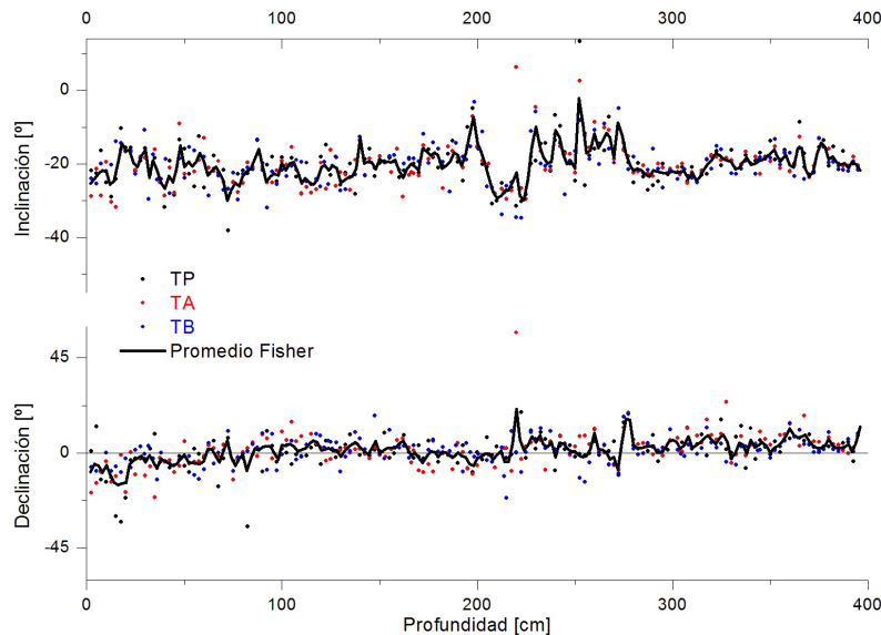
Figura 8. Inclinación I y declinación D. Los puntos indican los valores de I y D de la magnetización remanente estable. La línea indica el promedio Fisher de dichos datos.
