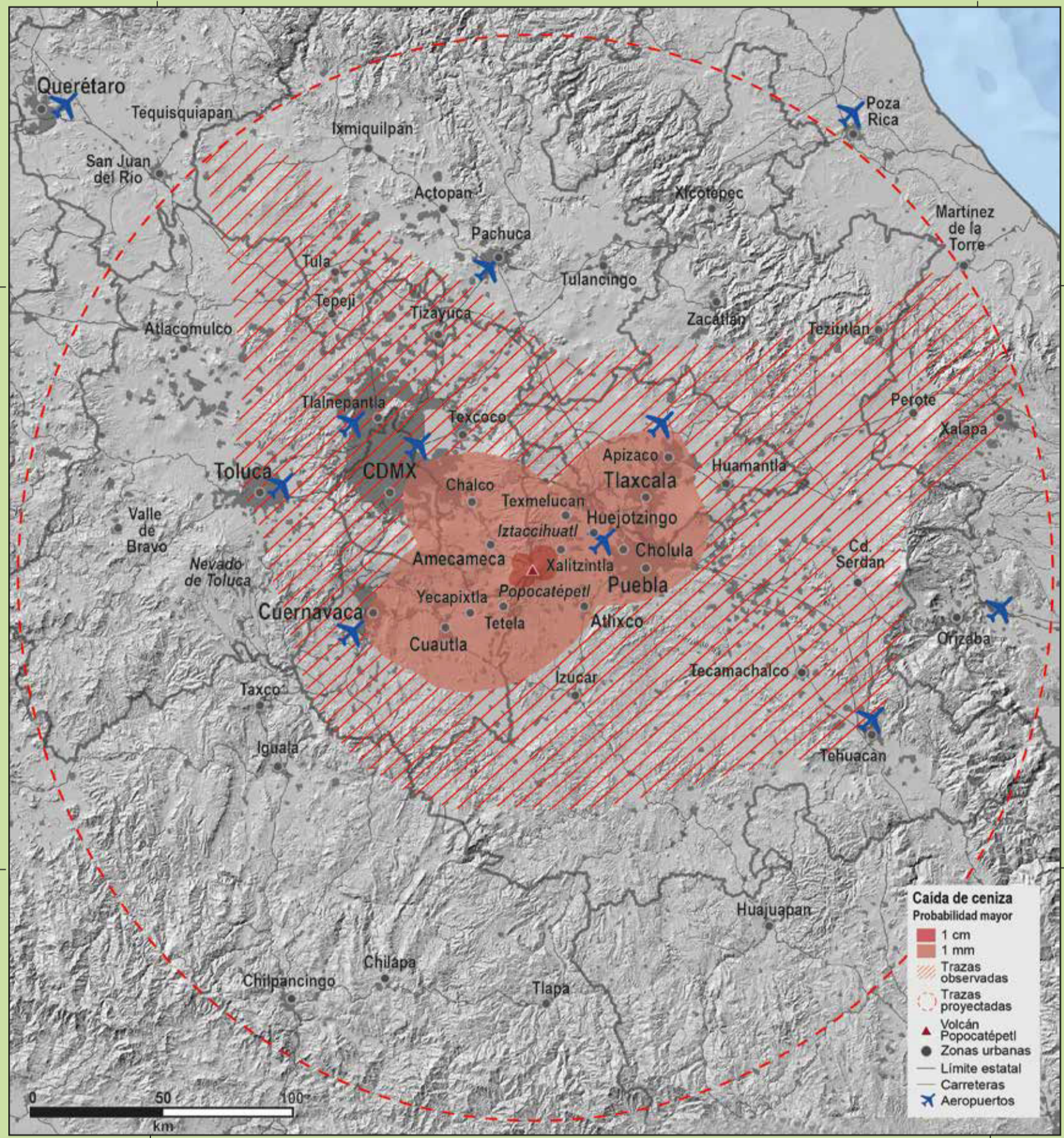
El escenario más probable (mapa en rojo), corresponde a las erupciones más frecuentes con columnas de ceniza menores a 10 km de altura. Los diferentes tonos en rojo muestran las áreas que pueden ser afectadas por caída de cenizas con espesores de 1 cm, 1 mm y trazas (menores a 1 mm).
