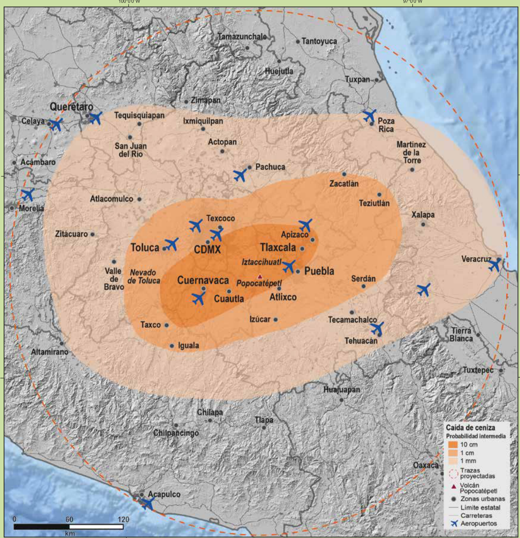
El escenario de probabilidad intermedia (mapa en naranja) muestra zonas en las que se puede depositar ceniza de erupciones con columnas con alturas entre 10 y 20 km. Los diferentes tonos en naranja indican áreas con caída probable de 10 cm, 1 cm, 1 mm y trazas.
